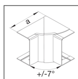
Coltar interior reglabil PC - ABS fara continut de halogen
